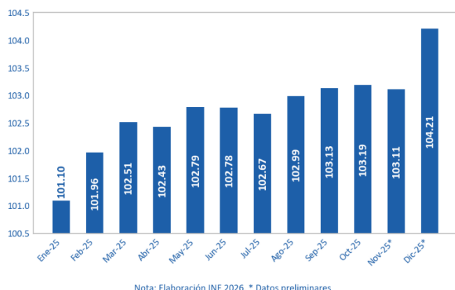
Gráfico 2. Índice General IPP enero –diciembre 2025 Base 2024 = 100.00 – Sección C
